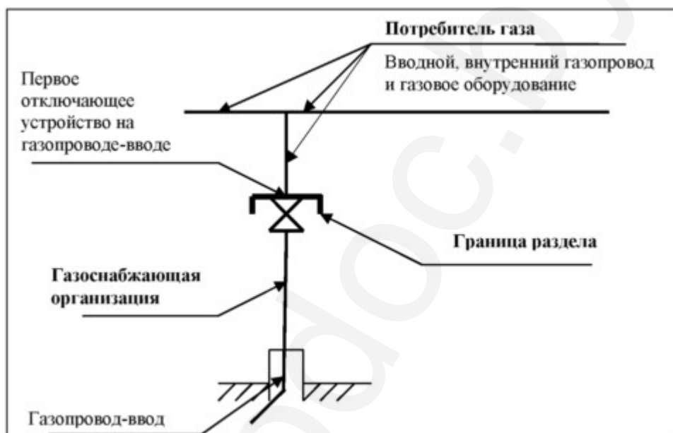
Примерная схема
