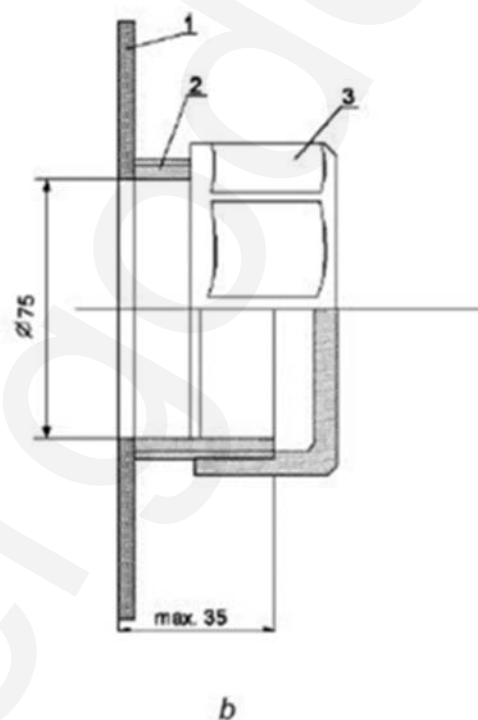
Рисунок Л.4 – Пример круглого входного отверстия с внутренним диаметром 75 мм с внутренней резьбой (a) и наружной резьбой (b)
