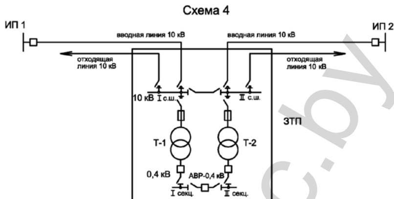
Рисунок 4 – Схема присоединения ТП 10/0,4 кВ, питающей потребителей категории 1
