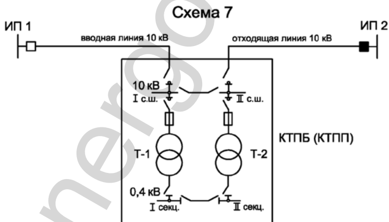
Рисунок 7 – Схема присоединения ТП 10/0,4 кВ, питающей потребителей категории 2
