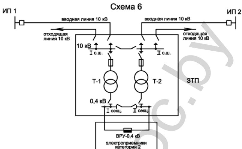
Рисунок 6 – Схема присоединения ТП 10/0,4 кВ, питающей потребителей категории 2
