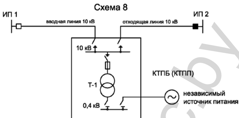
Рисунок 8 – Схема присоединения ТП 10/0,4 кВ, питающей потребителей категории 2
