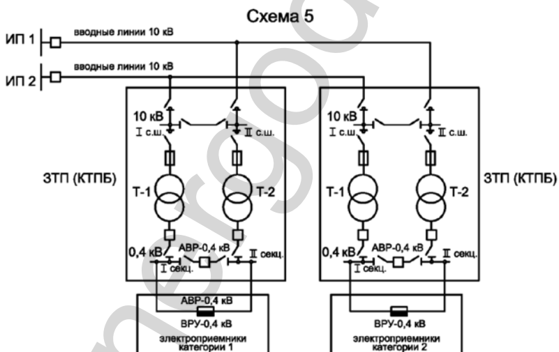
Рисунок 5 – Схема присоединения ТП 10/0,4 кВ, питающей потребителей категорий 1 и 2
