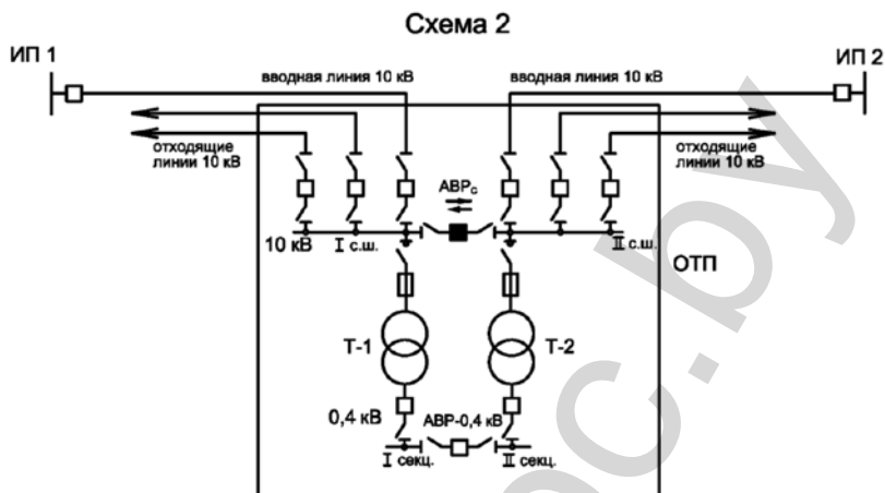
Рисунок 2 – Схема присоединения ТП 10/0,4 кВ, питающей потребителей категории 1
