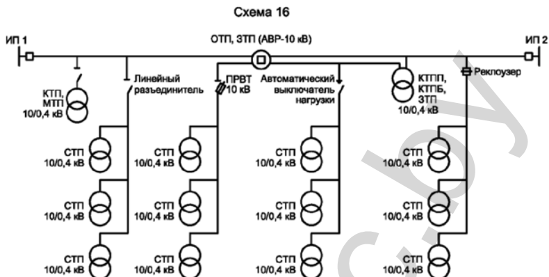
Рисунок 14 – Схема сети PC_{\text{стп}} с переносом источников трансформации (СТП 10/0,4 кВ) к потребителю в сельских населенных пунктах
