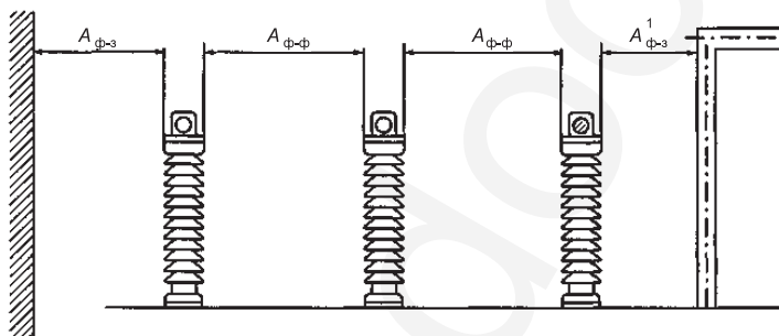
Рисунок 6.2.3 – Наименьшие расстояния в свету при жестких шинах между токоведущими и заземленными частями ( A_{\phi-3} , A_{\phi-3}^1 ) и между токоведущими частями разных фаз ( A_{\phi-ф} )
