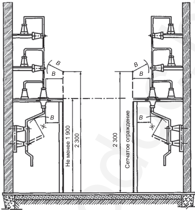
Рис. 6.2.16 – Наименьшие расстояния, мм, от неизолированных токоведущих частей в ЗРУ до сетчатых ограждений и между неогражденными неизолированными токоведущими частями разных цепей (см. таблицу 6.2.7)
