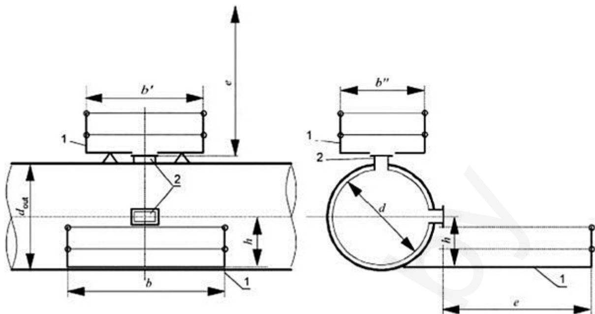
1 – рабочая площадка; 2 – измерительный порт; b , b' , b'' – длина рабочей зоны; d – внутренний диаметр газохода; d_{out} – наружный диаметр газохода; e – ширина рабочей зоны; h – минимальная высота свободной зоны над рабочей площадкой
