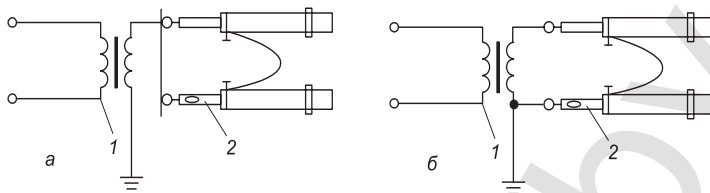
Рисунок 1 – Принципиальные схемы испытания указателя напряжения для проверки совпадения фаз по схеме согласного (а) и встречного (б) включения
