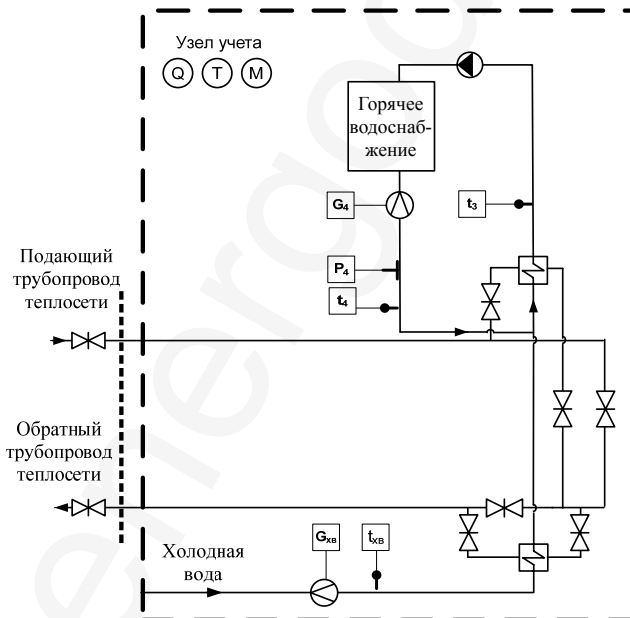
Рисунок 10 – Принципиальная схема горячего водоснабжения потребителей (ЦТП, ИТП)
