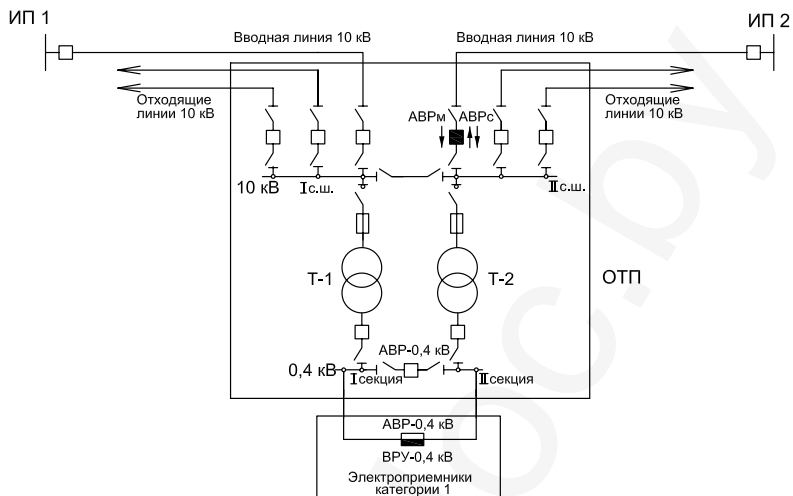
Рисунок 3 – Схема присоединения ТП 10/0,4 кВ, питающей потребителей категории 1
