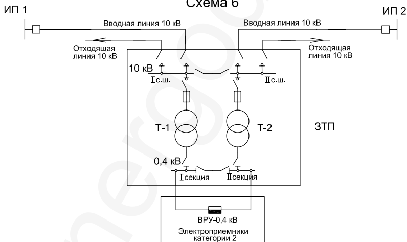
Рисунок 6 – Схема присоединения ТП 10/0,4 кВ, питающей потребителей категории 2
