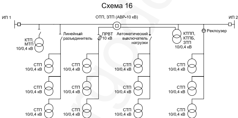
Рисунок 14 – Схема сети с переносом источников трансформации (СТП 10/0,4 кВ) к потребителю в сельских населенных пунктах
