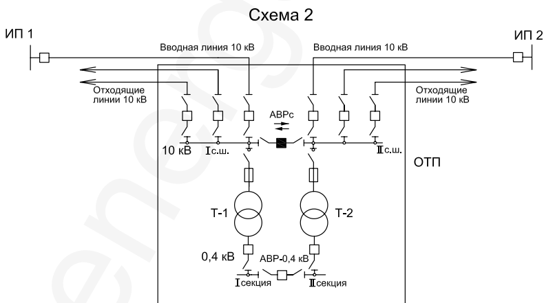
Рисунок 2 – Схема присоединения ТП 10/0,4 кВ, питающей потребителей категории 1
