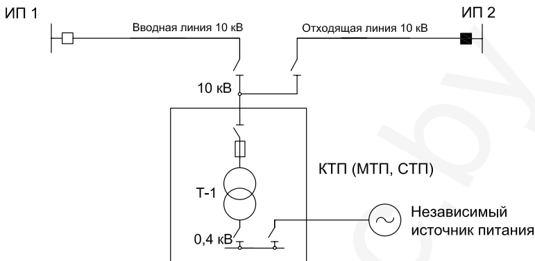
Рисунок 9 – Схема присоединения ТП 10/0,4 кВ, питающей потребителей категории 2
