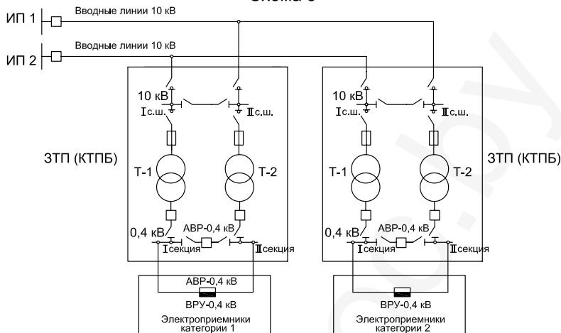
Рисунок 5 – Схема присоединения ТП 10/0,4 кВ, питающей потребителей категорий 1 и 2
