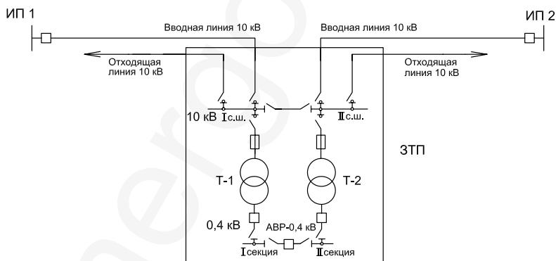
Рисунок 4 – Схема присоединения ТП 10/0,4 кВ, питающей потребителей категории 1
