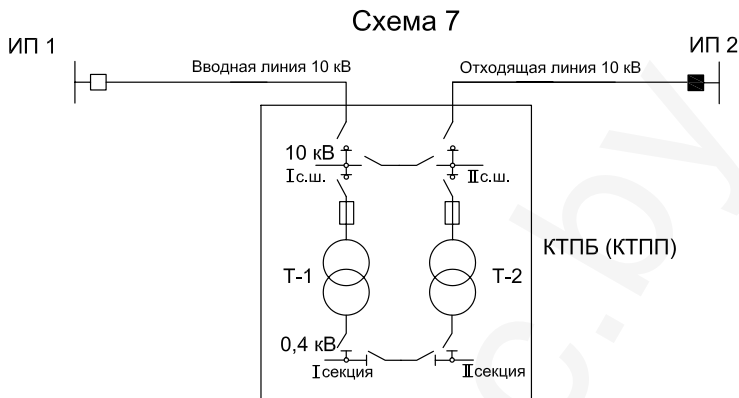
Рисунок 7 – Схема присоединения ТП 10/0,4 кВ, питающей потребителей категории 2
