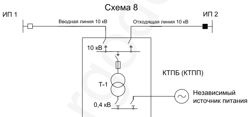
Рисунок 8 – Схема присоединения ТП 10/0,4 кВ, питающей потребителей категории 2
