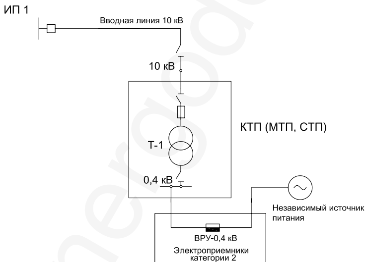
Рисунок 10 – Схема присоединения ТП 10/0,4 кВ, питающей потребителей категории 2
